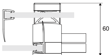
Przekrój dolnego systemu przesuwanego Cross-section of bottom sliding system Průřez spodním posuvným systémem
